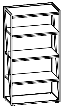
LMMC 80 800x430x1517
